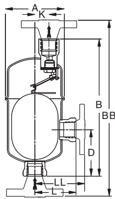
Model 22-AV and 13-AV
