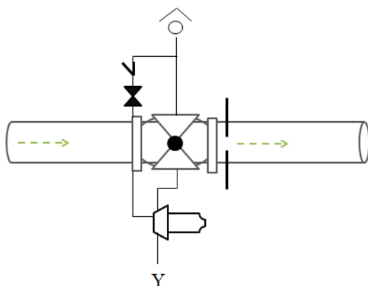
Figur 8. Avluftsventil
