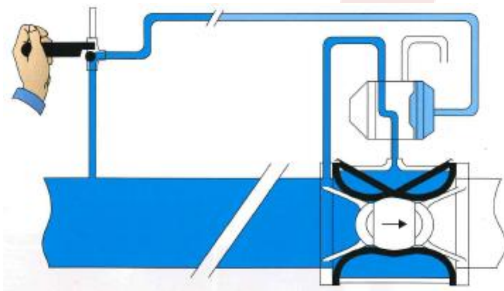
Figur 3. Manuell styrning
