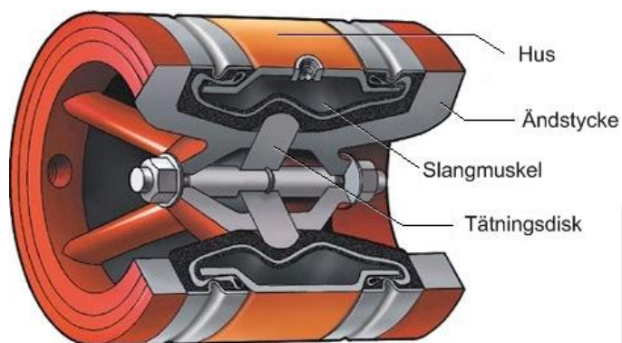
Figur 1. Design av ventil
